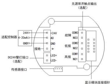
图 4-2 接线示意图
